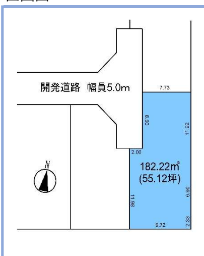
区画図
